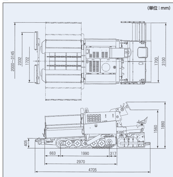
■ 外形図 / HB31C-5B
