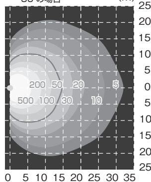
SL430LIDG 水平面照度分布図 (ルクス)
