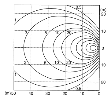
SLH440EG 水平面照度分布図 (ルクス)
