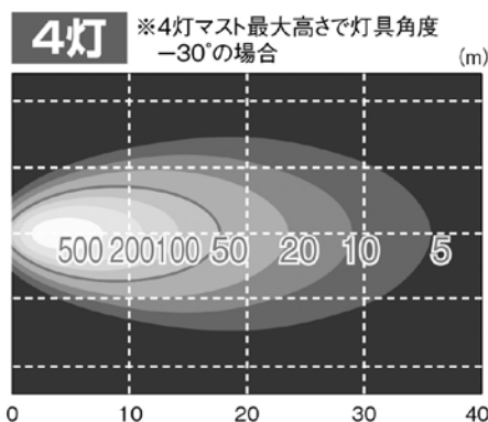
水平面照度分布図 (ルクス)
