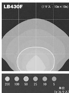
LB430F 照度測定分布図 (ルクス)
